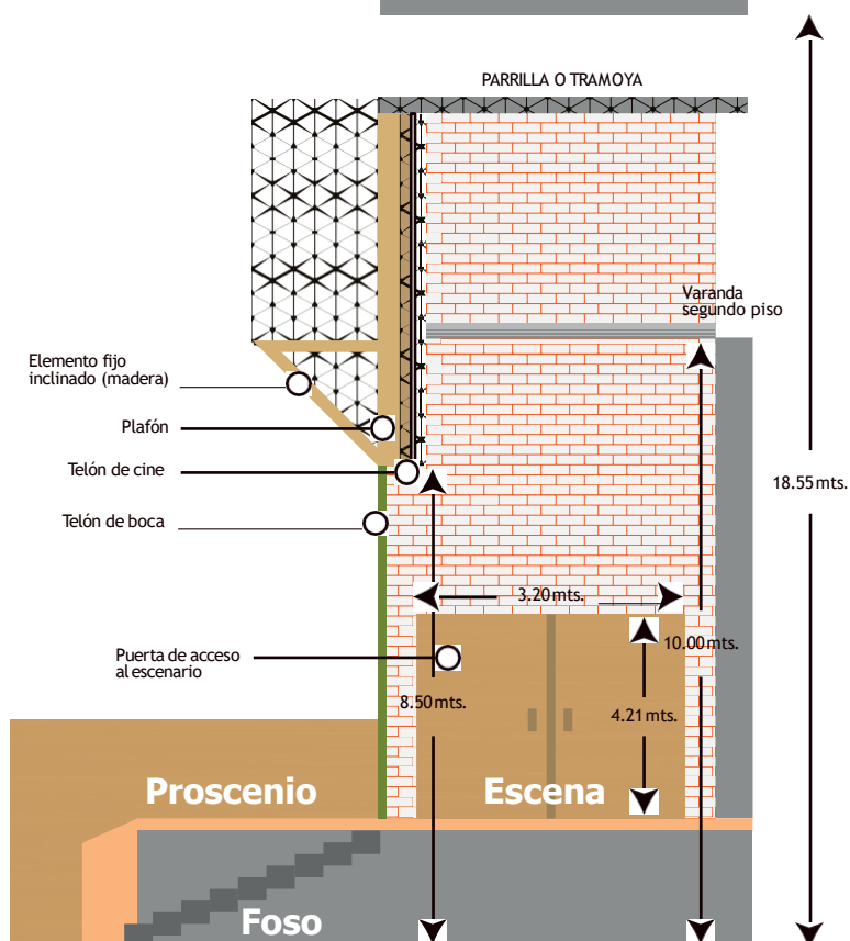
CORTE LONGITUDINAL ESCALA 1:75
