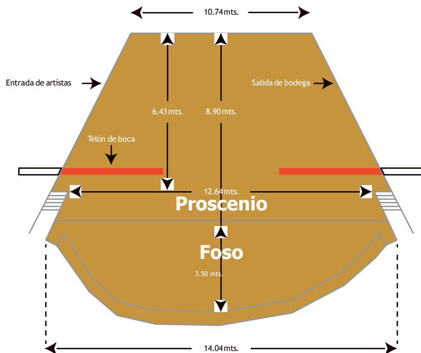
PLANTA ESCENARIO ESCALA 1:75
